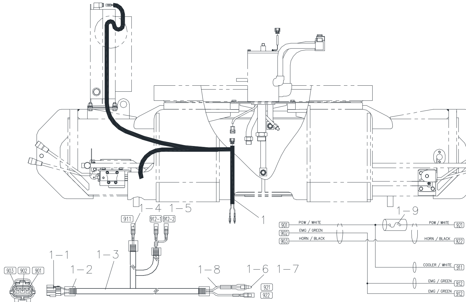
Fig. 8-1 SCS 1616 FRAME WIRING
