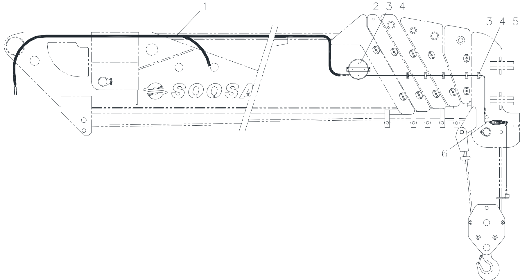
Fig. 8-3 SCS 1616 BOOM WIRING
